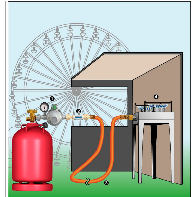
11-kg-Flaschenanlage im Freien bzw. im Marktstand etc. mit Schlauchleitung länger als 40 cm
