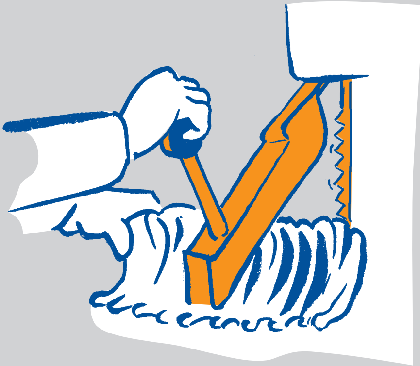
Bandsäge mit Andrückvorrichtung
